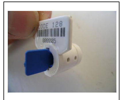
Art: TWISTSEAL Precinto de plástico con alambre grabado con láser Permite código de barras
