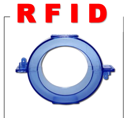
Art: CONNECTIONLOCK RFID MEDIDAS ART 311: para DN20 (3/4") ART 312: para DN20 (3/4") Union reforzada ART 313: para DN25 (1") ART 314: para DN40 (1 1/2") RFID UHF -HF/NFC
