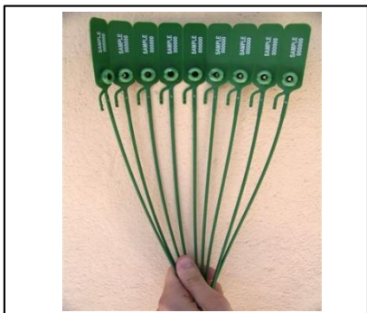
Art: JUPITER SEAL Precinto de plástico con mecanismo de cierre metalico Impresión con transferencia de tinta 2 x 315 mm 2 x 425 mm con o sin abertura rápida cola cilíndrica lisa
