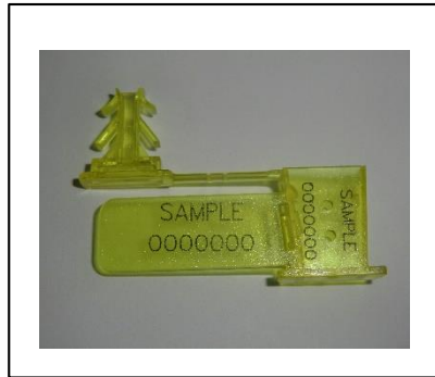
Art: ANCORFLAG Precinto de plástico grabado con láser. Permite código de barras
